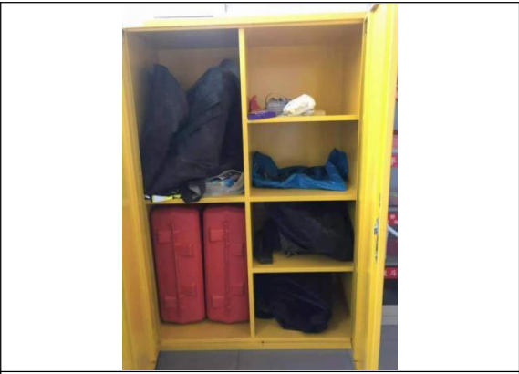
雨水排口及污水排口充气式封堵气囊
